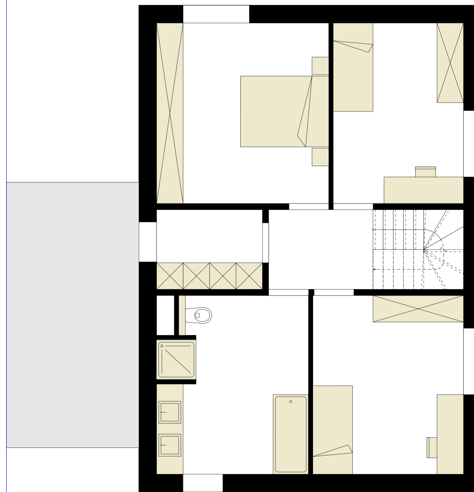
Niveau +1
