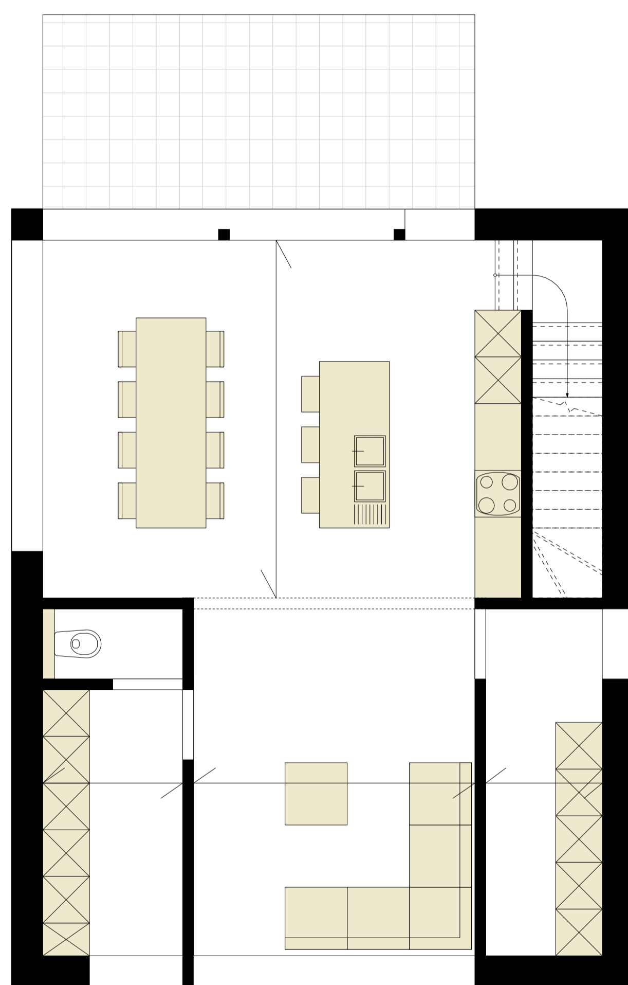
Niveau +0
